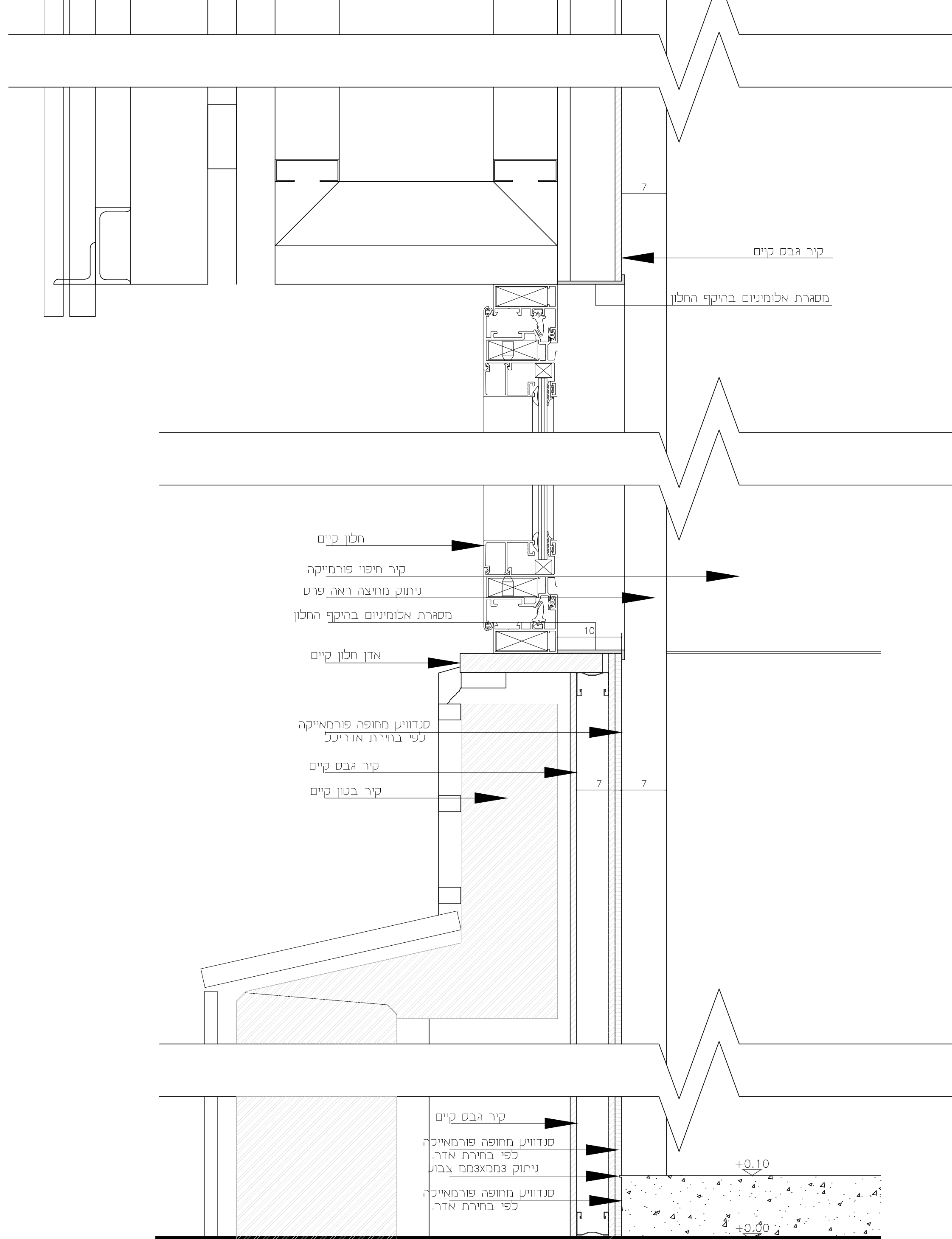
חתך דרך קיר חיצוני בעמדת עירווי
