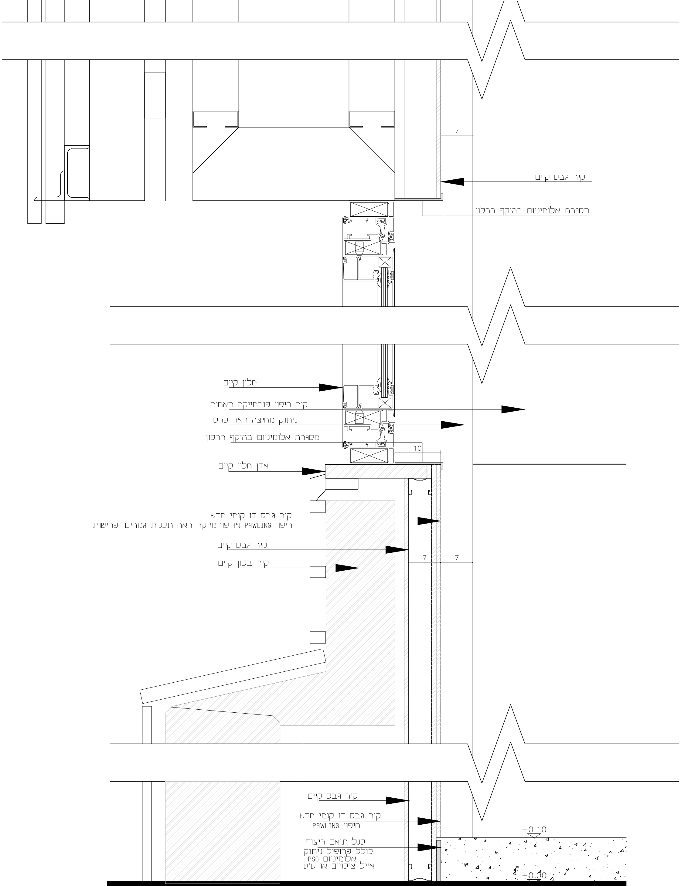
חתך דרך קיר חיצוני בעמדת השהייה
